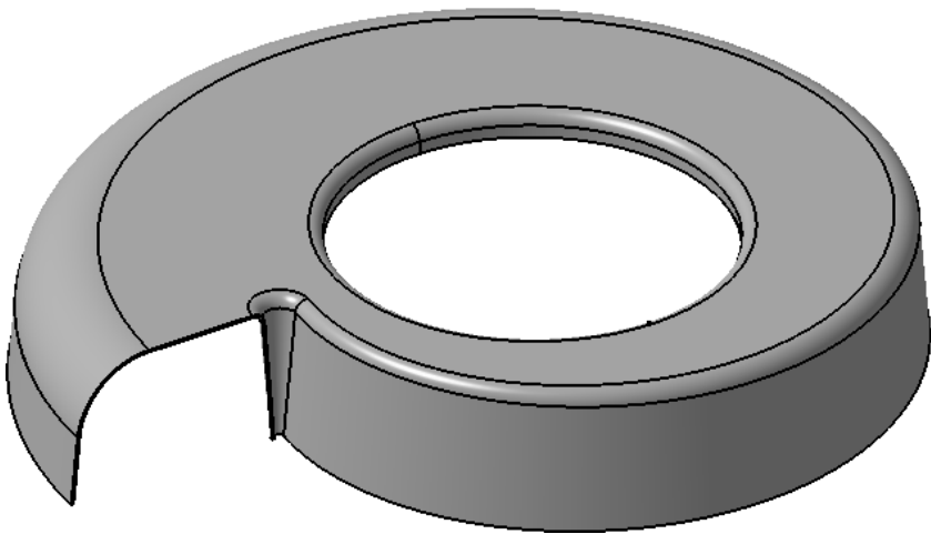
Isometric view Scale: 1:3
