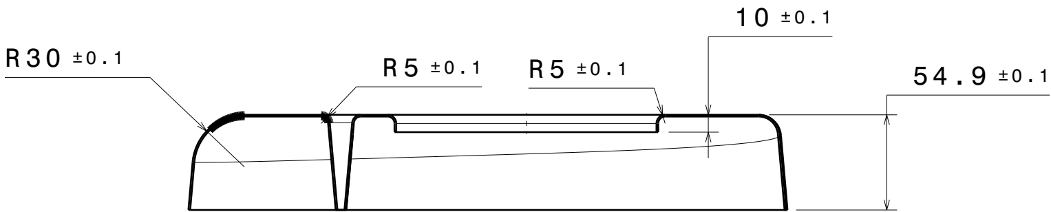
Section view A-A Scale: 1:3
