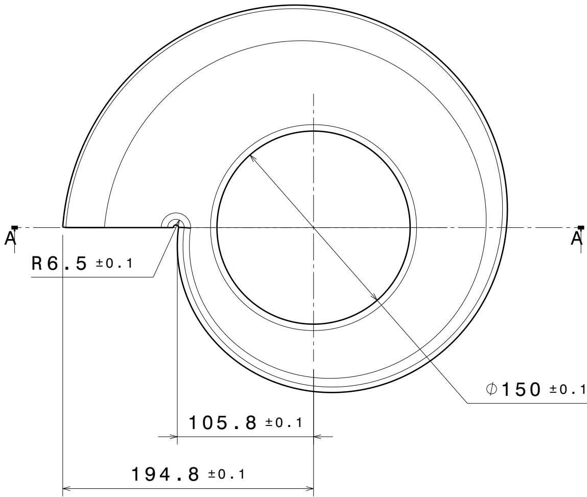
Top View Scale: 1:3
